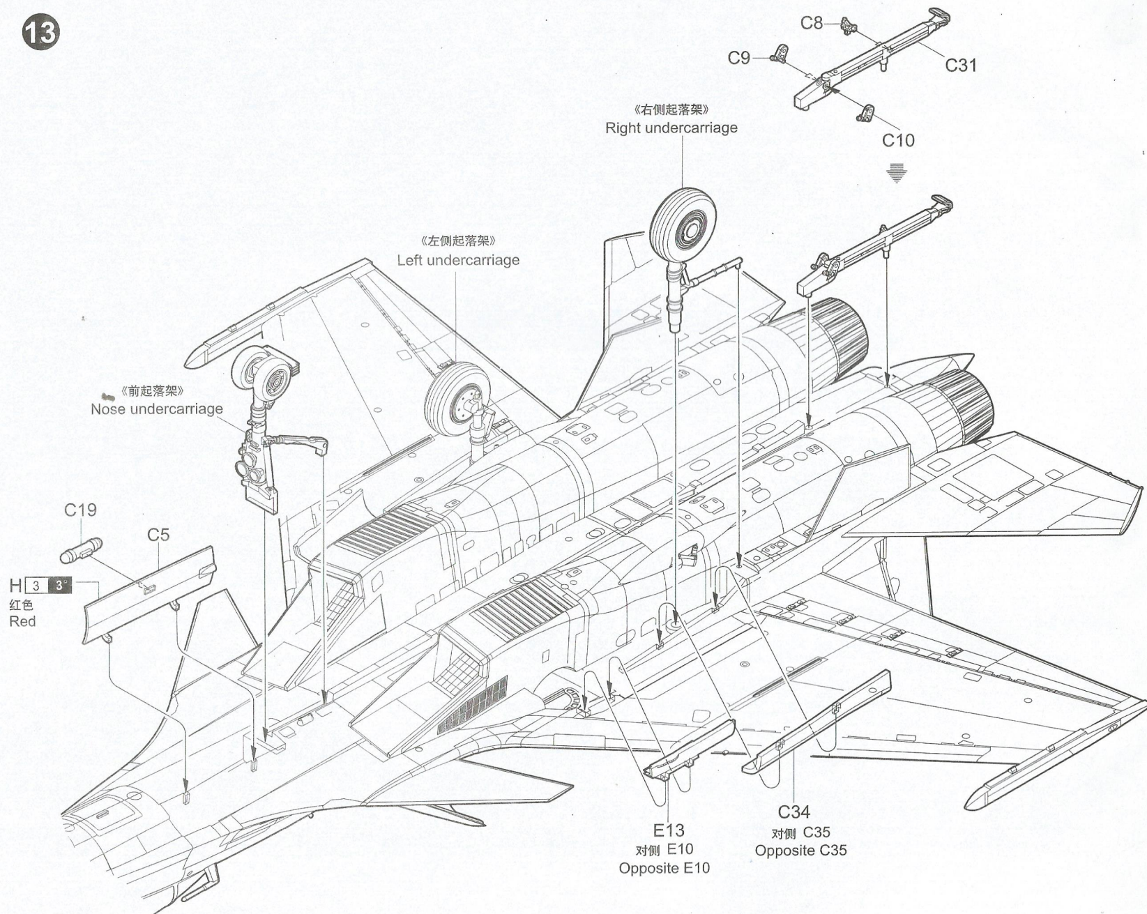
《右侧起落架》 Right undercarriage
