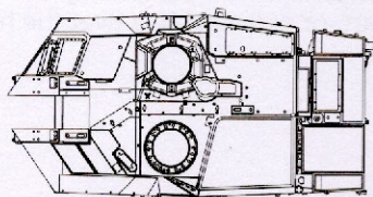
TURRET
