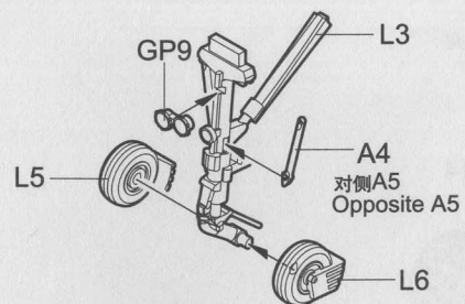
《前起落架》 Front undercarriage
