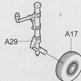
《右侧主起落架》 Right main undercarriage
